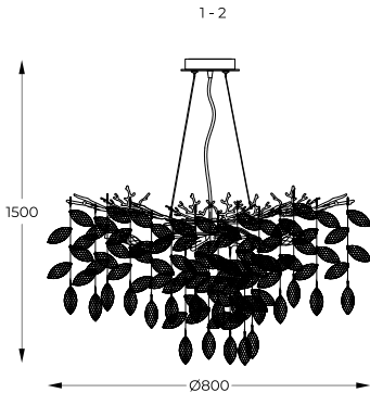
2. CINDY | Pendant lamp MD4115-1-ECN 10 x G9 MAX 3,5W metal chrome body glass shade
